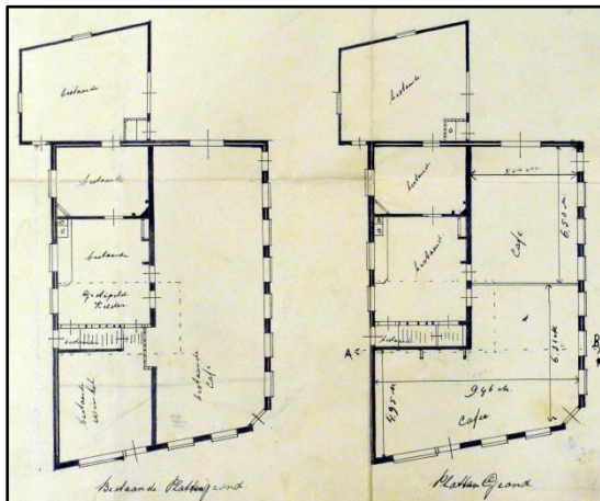
Verbouwing 1931, links bestaand, rechts vernieuwd..
