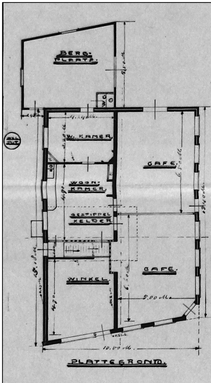
Plattegrond van de benedenverdieping.
