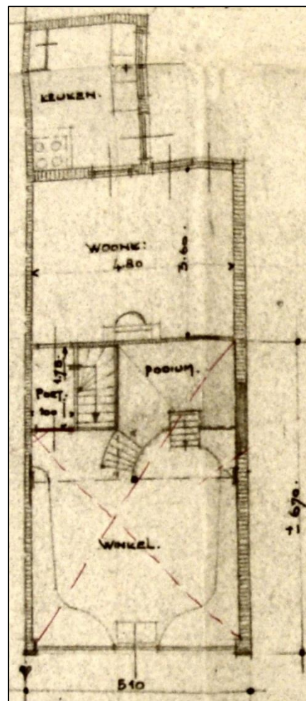
Tekeningen bij de aanvraag voor de verbouwing in 1957.
